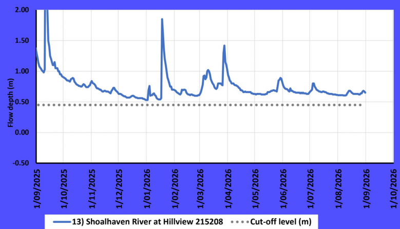
13. Shoalhaven R at Hillview (site ID 215208) Min. level = 0.45 m.
