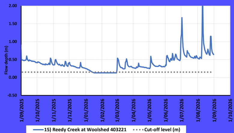
15. Reedy Creek (site ID 403221) Min. level = 0.22 m.
